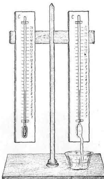
Рис. 12. Стационарный психрометр
