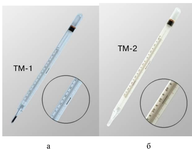
Рис.11. Термометры: а – максимальный, б - минимальный
